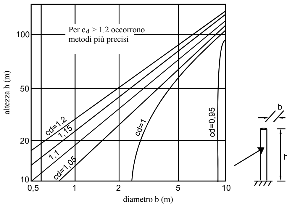
Fig. C.7.11 (b) - Ciminiere in acciaio, saldate, con rivestimento interno
