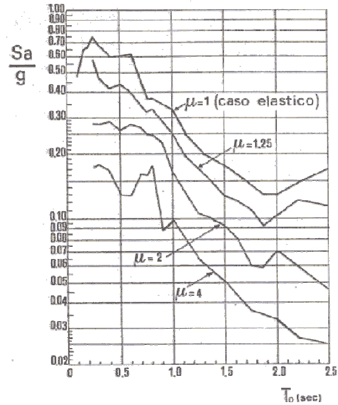
Pseudo accelerazione spettrale per diversi valori del fattore di duttilità
