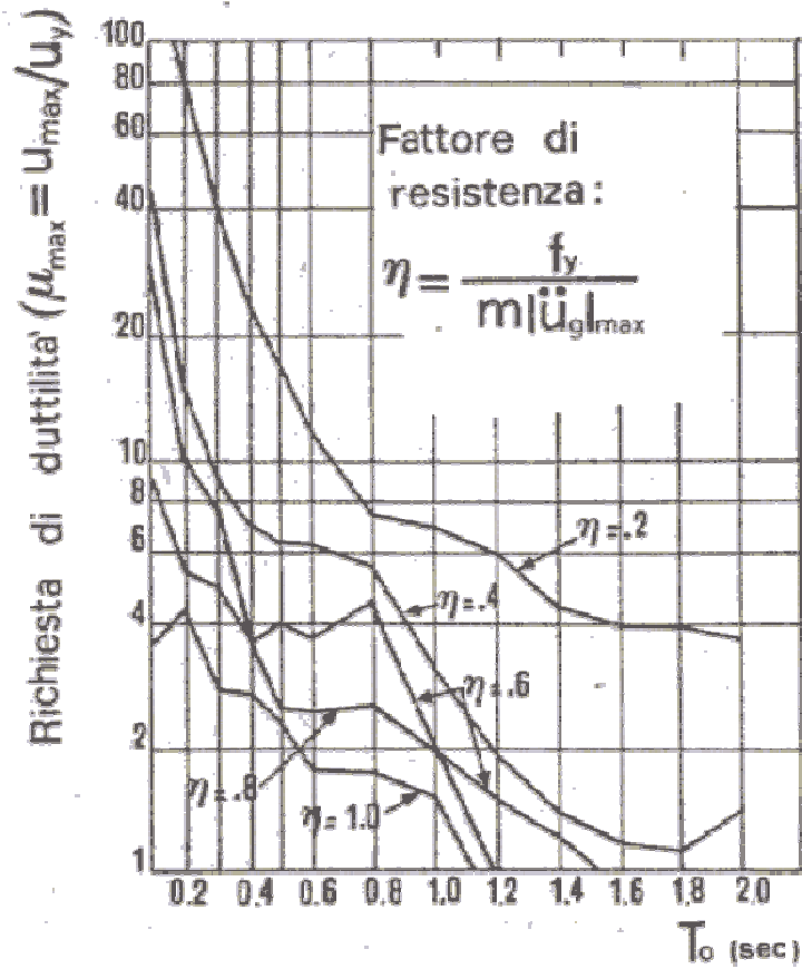
Richiesta di duttilità per diversi valori del fattore di resistenza
